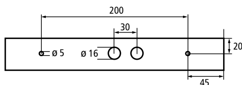
Bohrabstände
